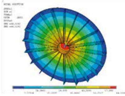
Thermal FEA
